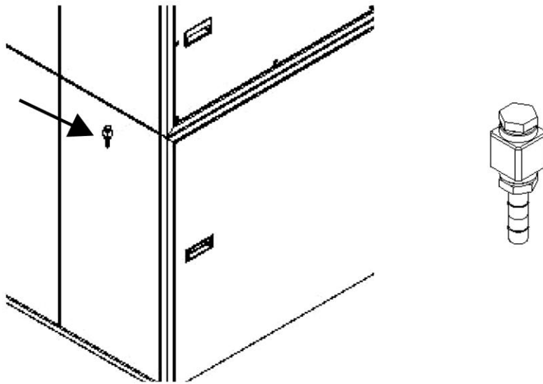
Afb. 28: Aansluiting persluchtvoorziening
