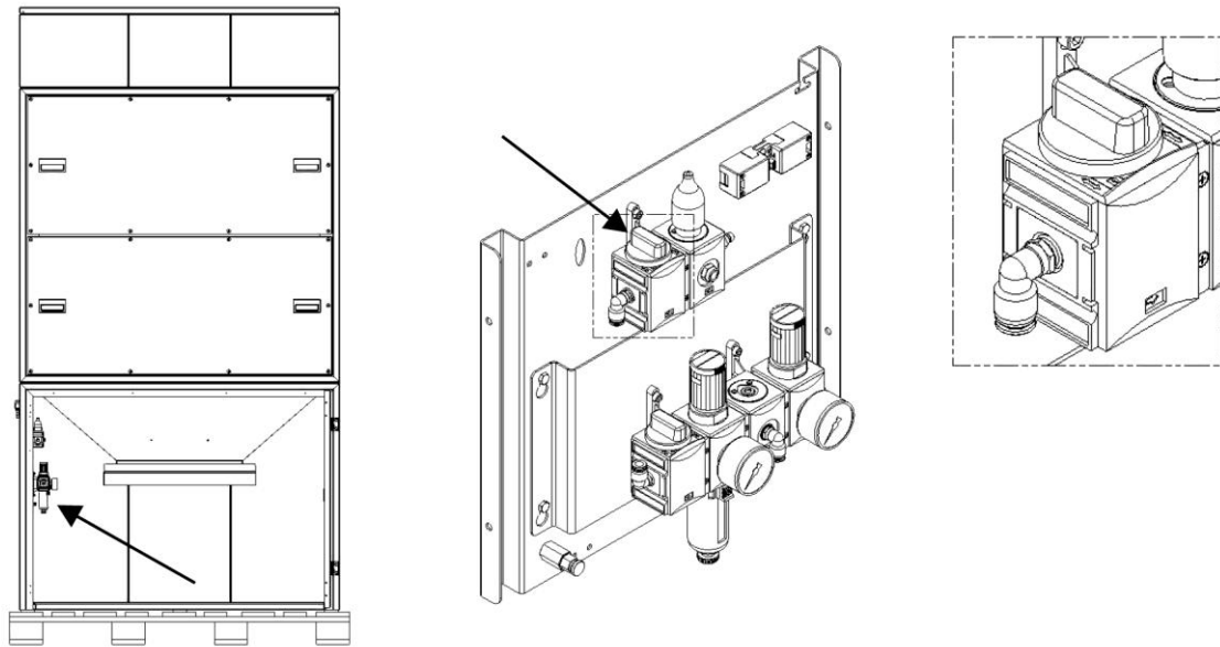
Afb. 14: Reductieventiel stofverzamelreservoir
