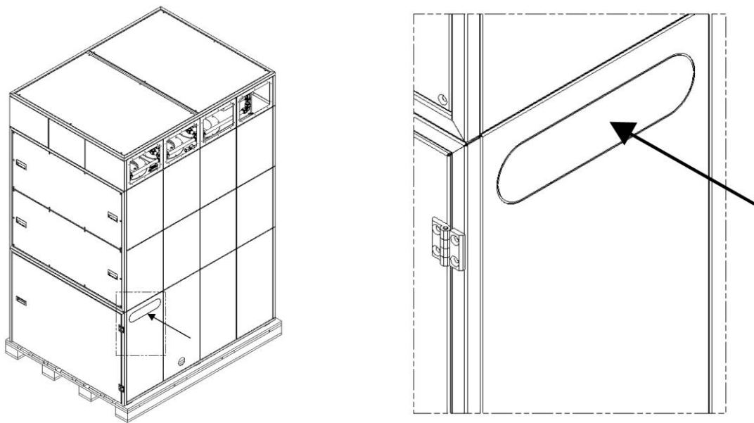
Afb. 13: Geperforeerde plaat
