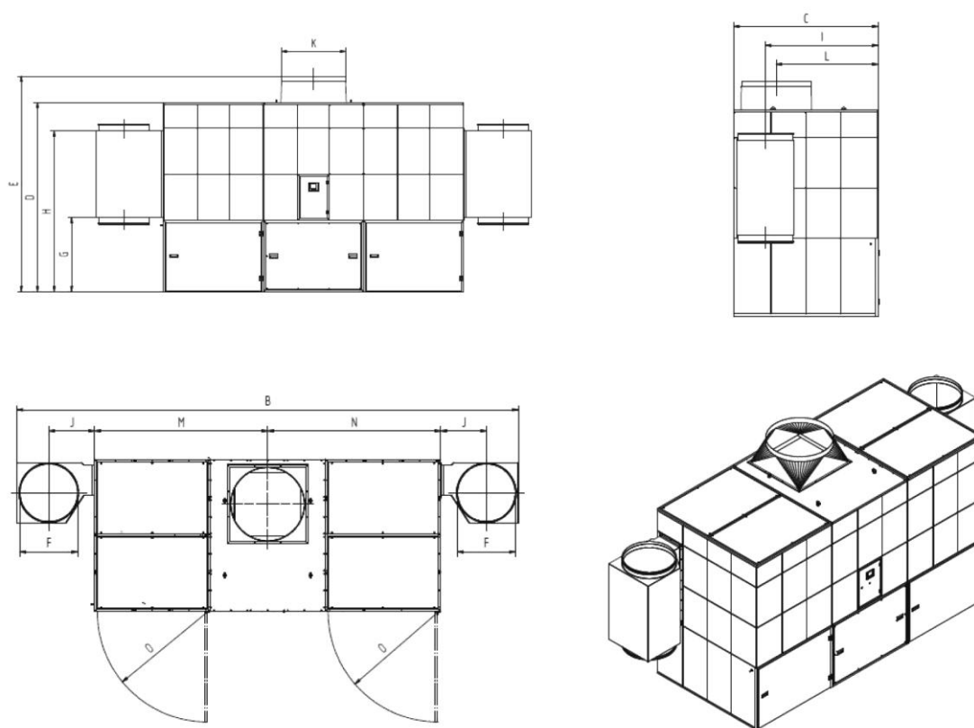
Afb. 77: Maatblad 34160
