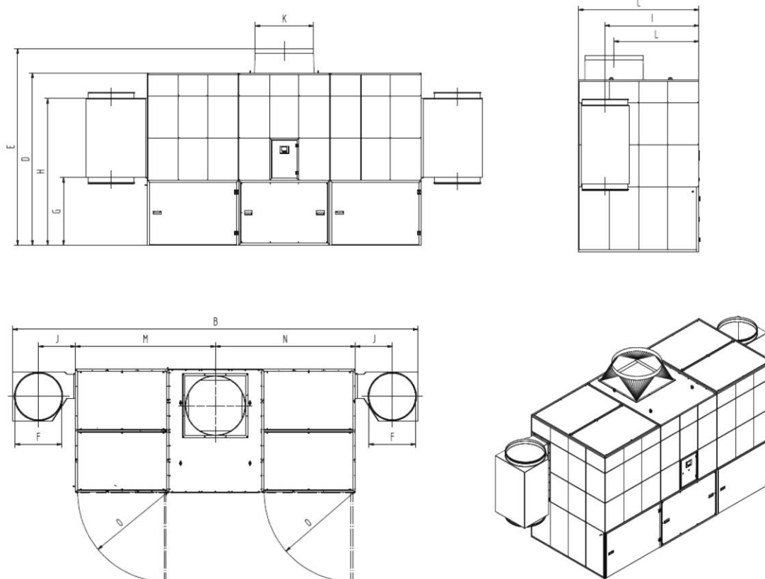
Afb. 80: Maatblad 34240 + 34270
